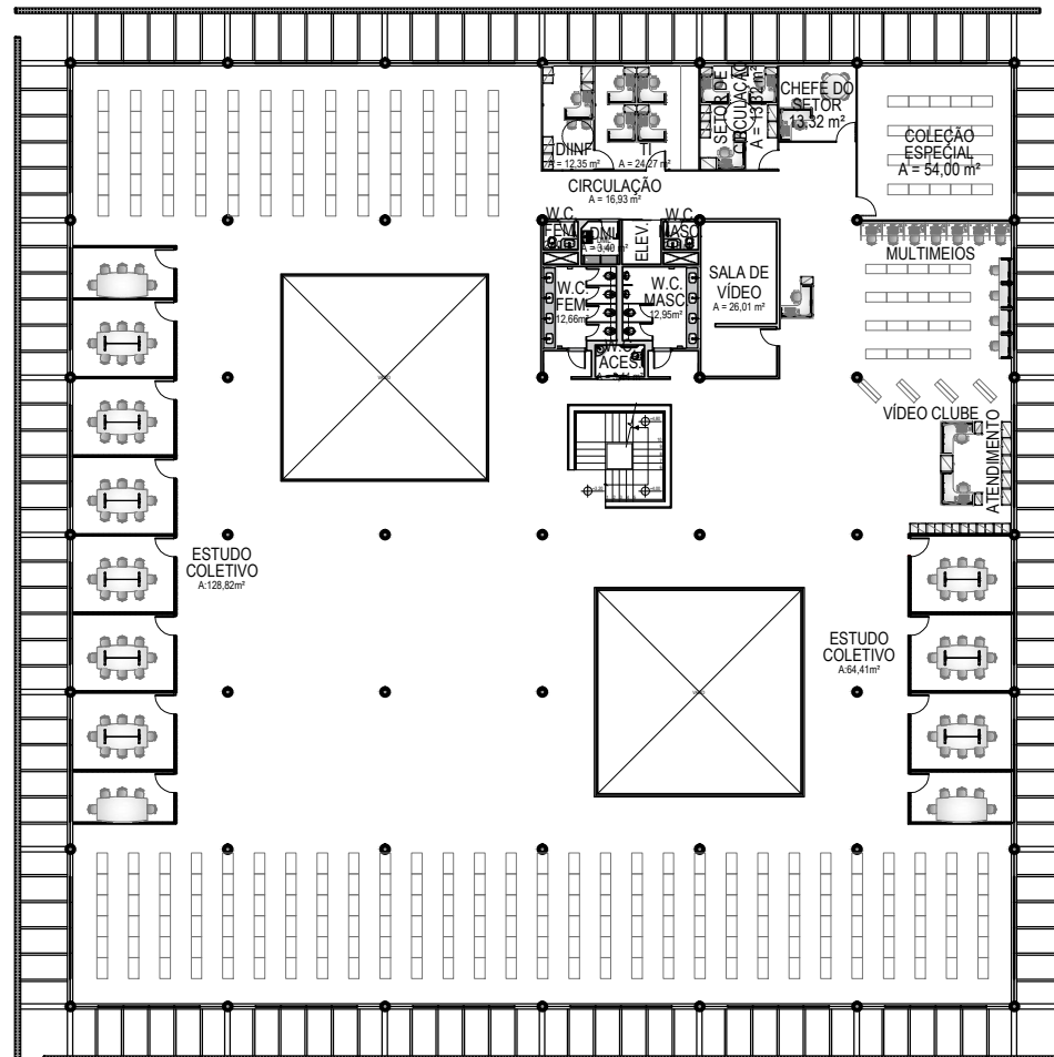
02 PLANTA LAYOUT 1º PAVIMENTO 3CSM - BIBLIOTECA ESC.: 1/400
