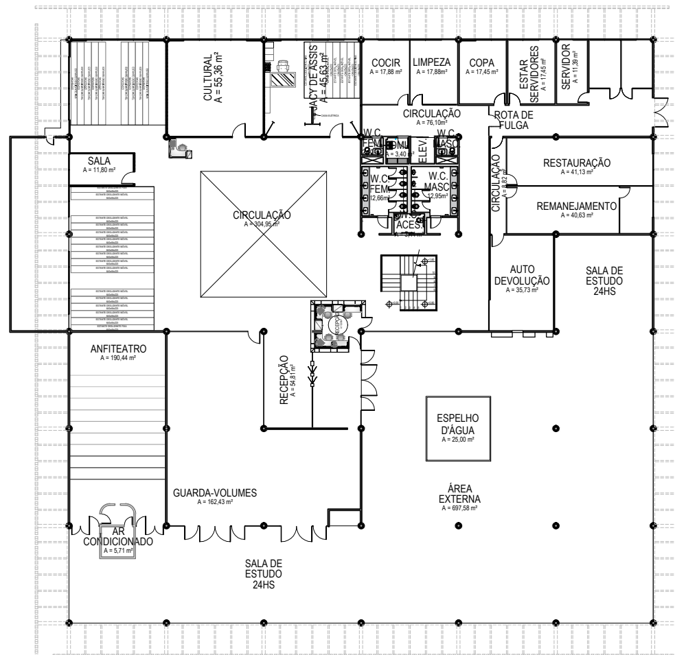
01 PLANTA LAYOUT TÉRREO 3CSM - BIBLIOTECA ESC.: 1/400
