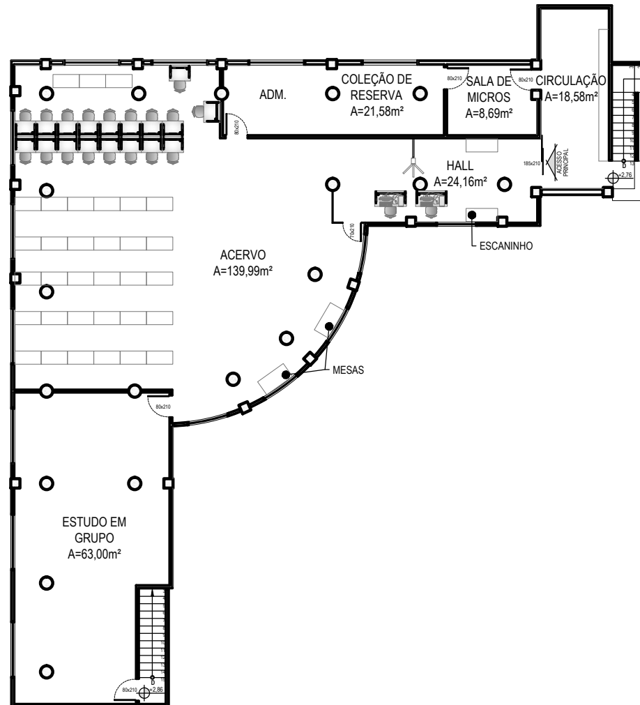
01 PLANTA LAYOUT PAV. SUPERIOR 1HEF - BIBLIOTECA ESC.: 1/200
