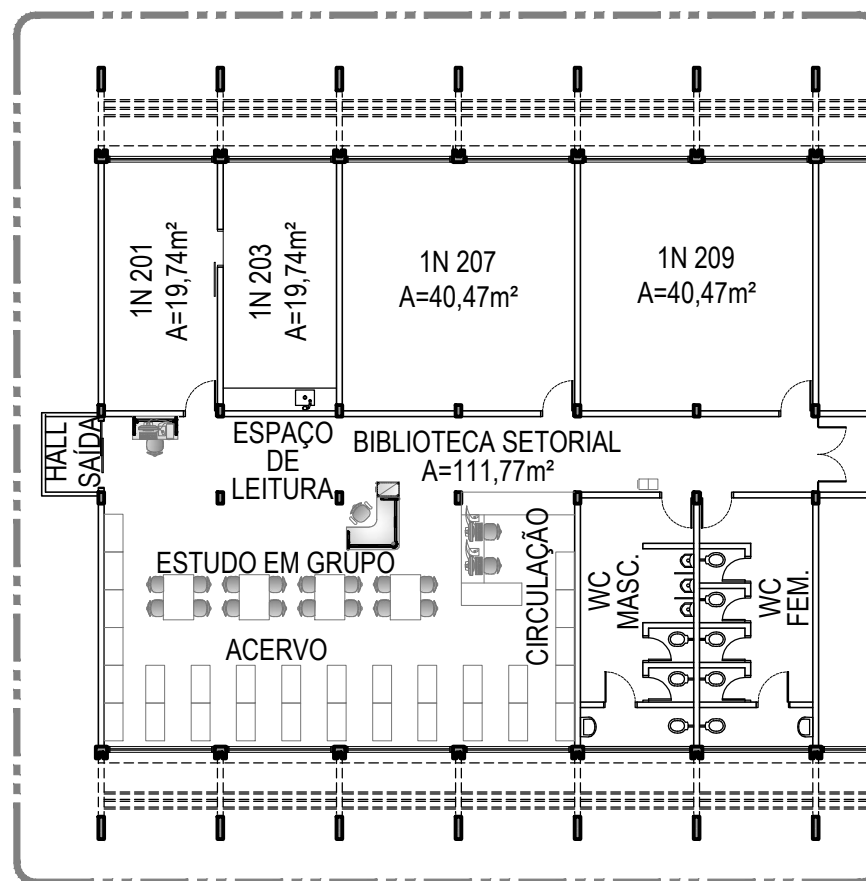
01 PLANTA LAYOUT BIBLIOTECA 1NEF - PAVIMENTO TÉRREO ESC.: 1/200
