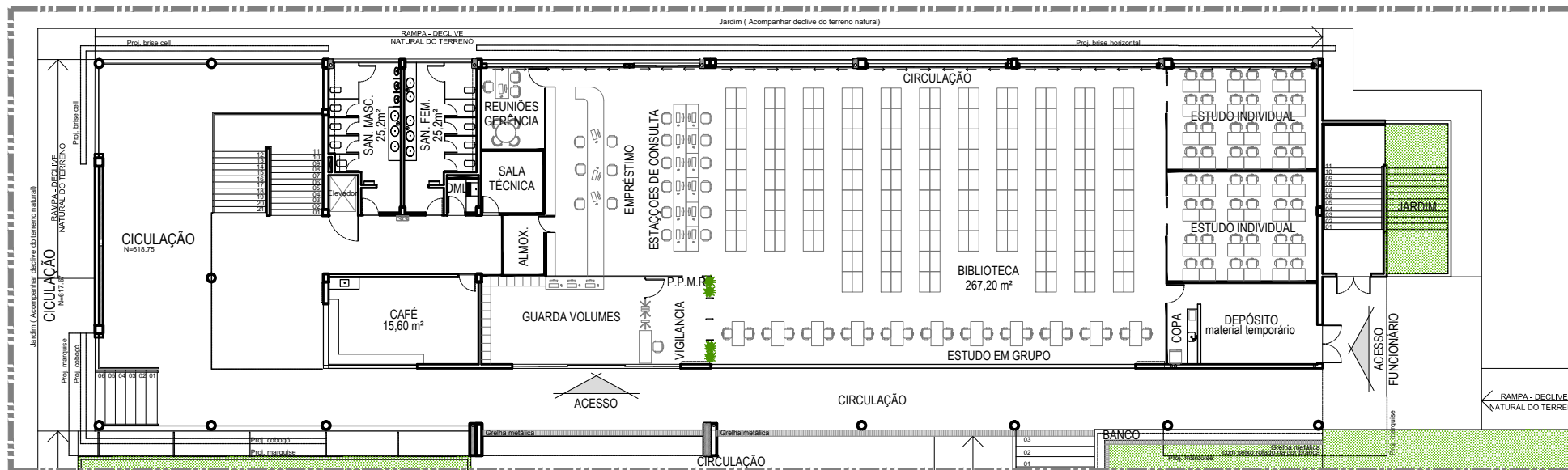
01 PLANTA DE LAYOUT 1CPL - BIBLIOTECA ESC.: 1/300
