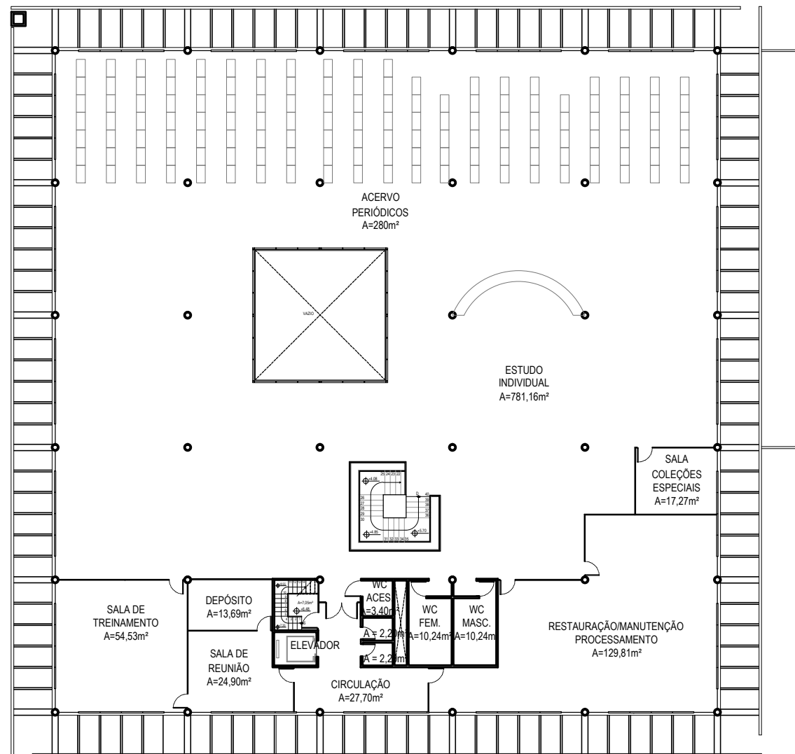
03 PLANTA DE LAYOUT 2º PAVIMENTO 4GJU-BIBLIOTECA ESC.: 1/300
